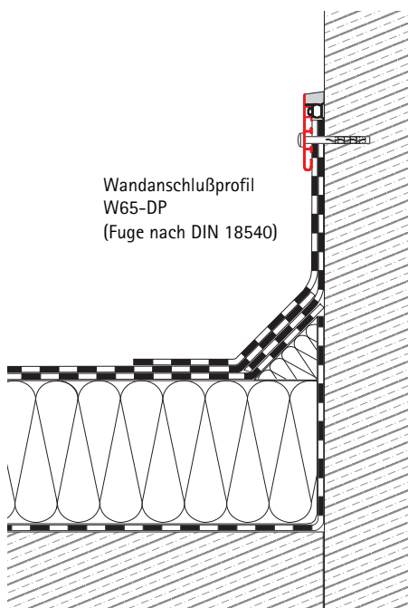
Terrassen- Wandanschlußprofil TW150
