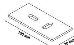
Thermostopp-Platte (d=5mm) 2x Stanzung 10,5 x 30 mm
