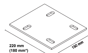
Thermostopp-Platte (d=5mm) 4x Stanzung 12,5 x 30 mm
