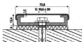
GW 225 / GW 275 mit Abdeckprofil und Thermostopp-Platte
