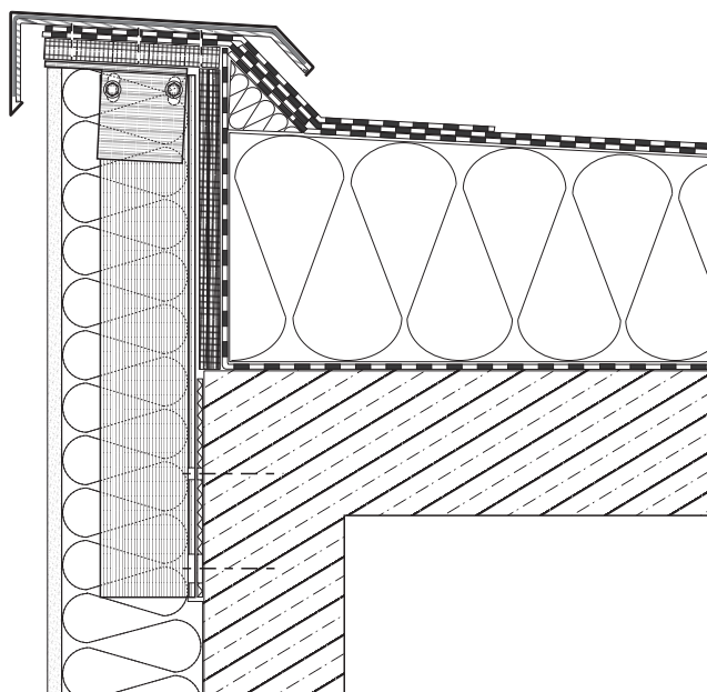
MAG 4K mit Rillenhalterprofil Dachrandaufbau fassadenseits
